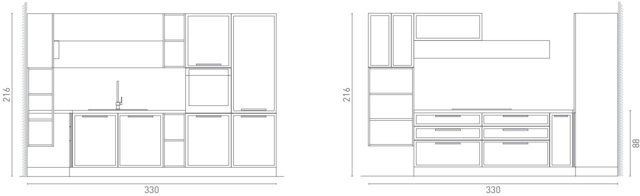
Basi Base units / Éléments bas / Unterschränke / Muebles bajos / Основания / Szafki dolne
