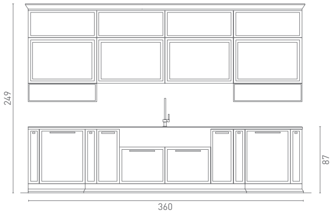
Basi e Pensili Base and wall units / Éléments bas et Éléments hauts / Unterschränke und Hängeschränke / Muebles bajos y Colgantes / Основания и навесные шкафы / Szafki dolne i Szafki wiszące
