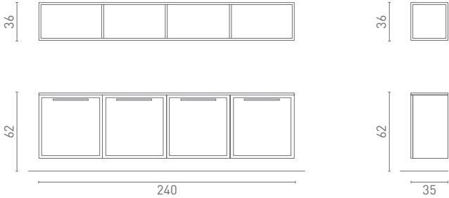
Pensili Wall units / Éléments hauts / Hängeschränke / Colgantes / Навесные шкафы / Szafki wiszące
