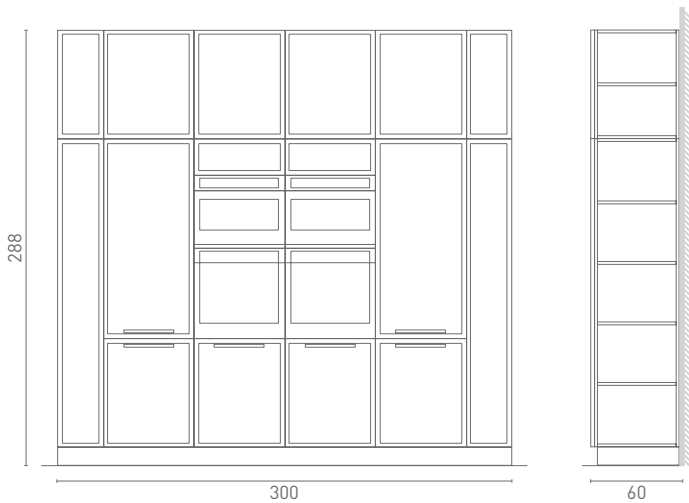
Colonne Tall units / Armoires / Hochschränke / Columnas / Колонны / Stupki
